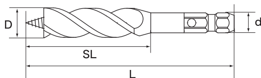
サイズ:D 全長:L ネジ丈:SL 軸径:d (単位:mm)
